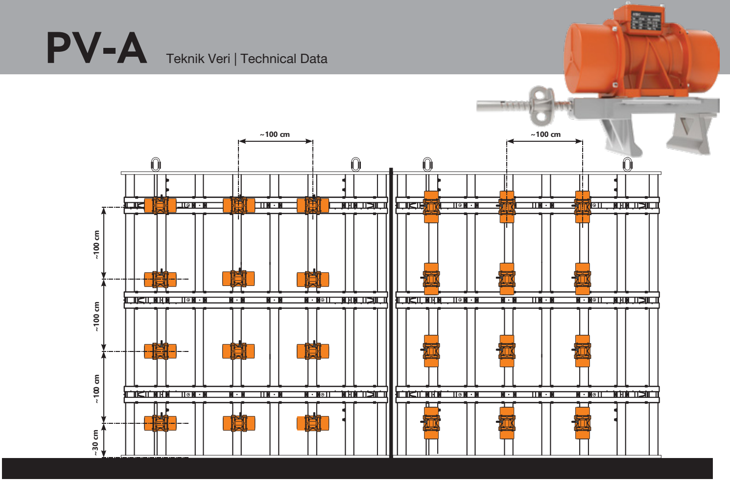
Şekil 1: Plywood Ahşap ve Çelik Beton kalıplarına sistematik vibrasyon motoru yerleştirme Figure 1: Placement of systematic vibration motors on wooden and steel concrete moulds
