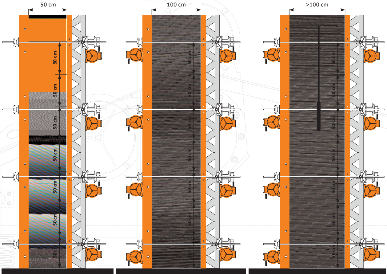
Şekil 2: PV-A serisi vibrasyon motorunun etkili sıkıştırma derinliği. Figure 2: Placement of PV-A series vibration motors efficient depth of compacting.
