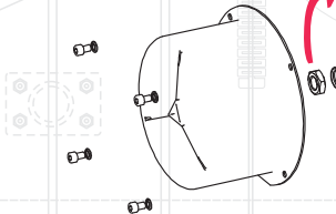
Sac delikli ağırlıklar Frontal Fixing Weights
